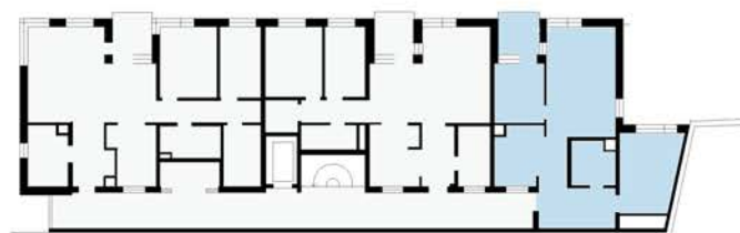
Våningsplan
